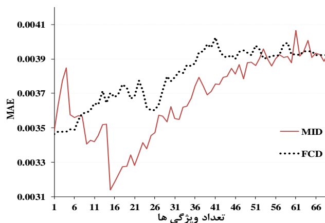
شکل ۲. استفاده از مدل RBF و ویژگی‌های اولویت‌بندی شده با روش‌های MID و FCD برای پیش‌بینی روزانه شاخص بورس
