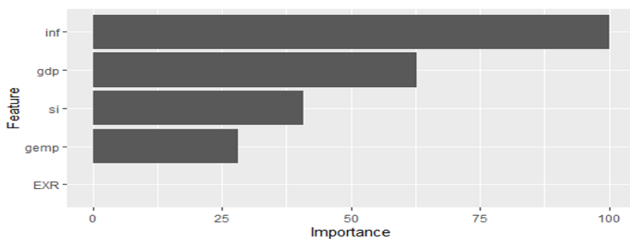
شکل ۵. درصد اهمیت مدل ستیغی منبع: یافته‌های محقق
