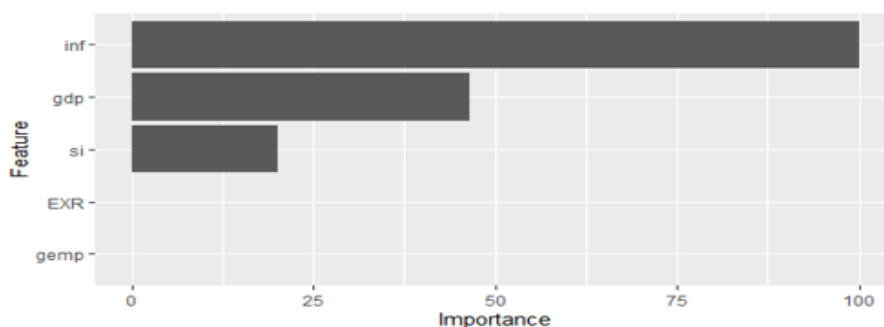
شکل ۶. درصد اهمیت مدل الستیک نت منبع: یافته‌های محقق
