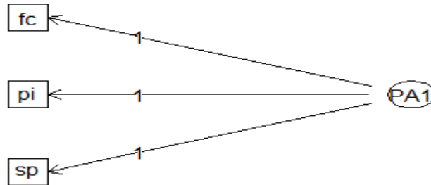
شکل ۳. تحلیل عاملی اکتشافی
