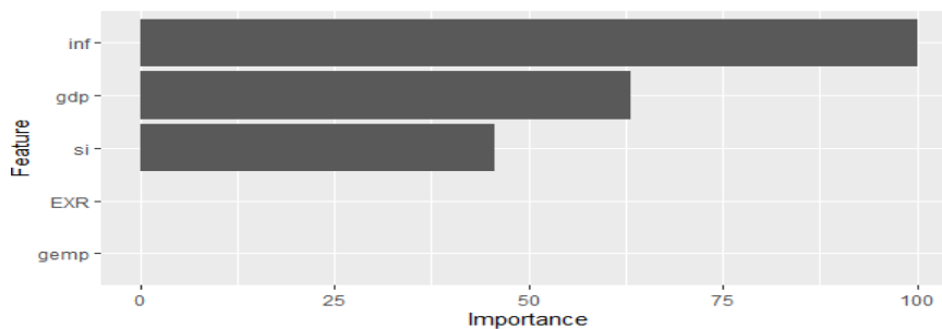
شکل ۴. درصد اهمیت مدل لاسو
