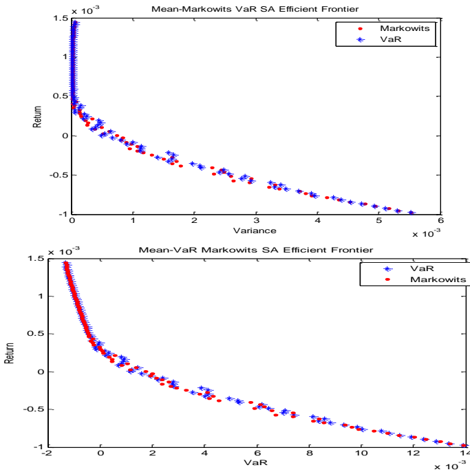
نمودارهای ۱۶ و ۱۷. مرزهای کارایی الگوی مارکویتز و الگوی ارزش در معرض ریسک پارامتریک با استفاده از تابع محلی fmincon
