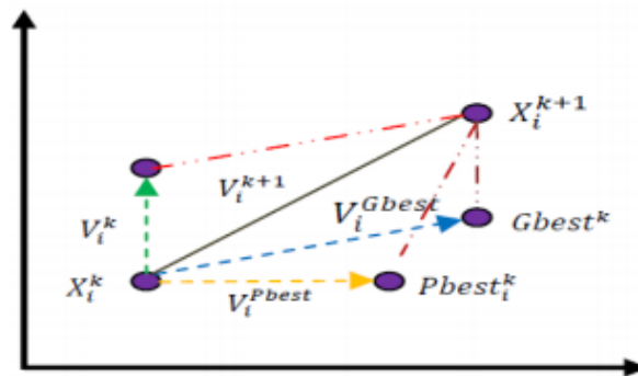
شکل ۲. فرآیند تغییر موقعیت ذرات در الگوریتم بهینه‌سازی حرکت تجمعی ذرات
